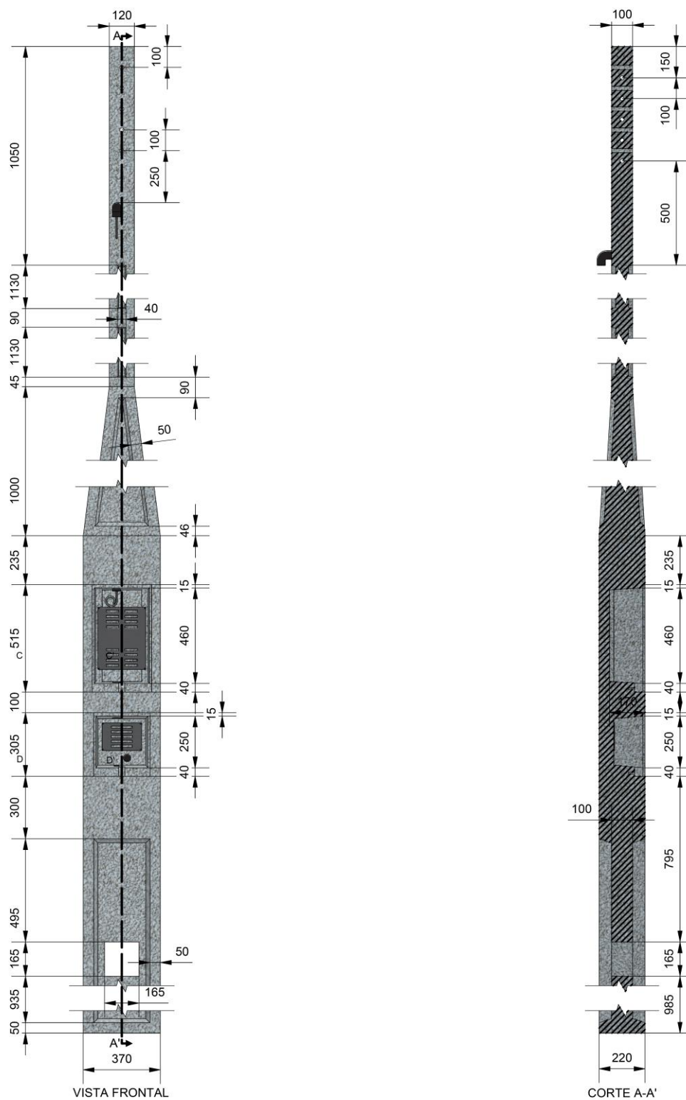
Figura 2 - Poste com uma medição e proteção incorporada – Vista frontal e corte lateral
