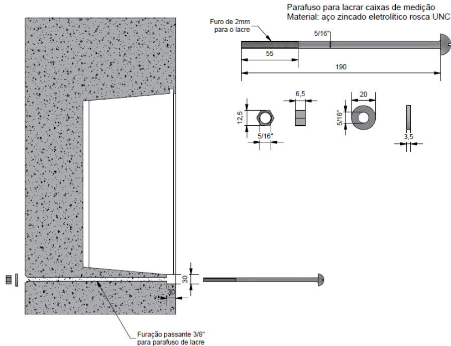
Figura 6 - Detalhe de fixação da tampa da medição e proteção
