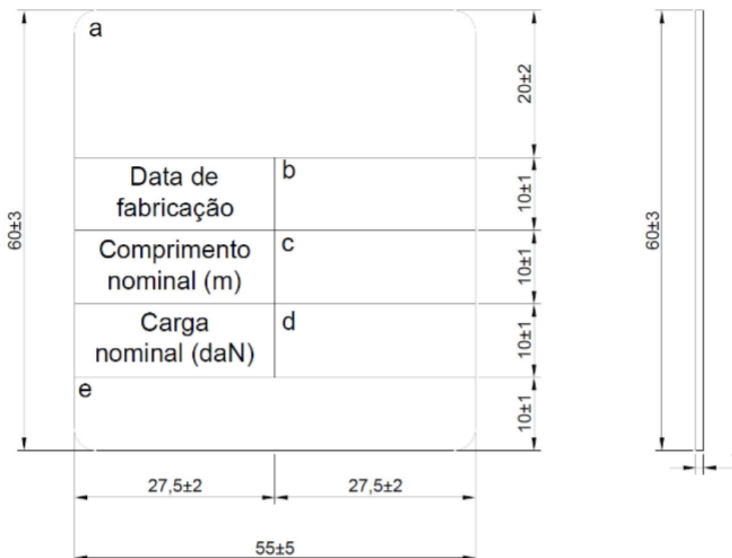
Figura 7 - Identificação na placa metálica
